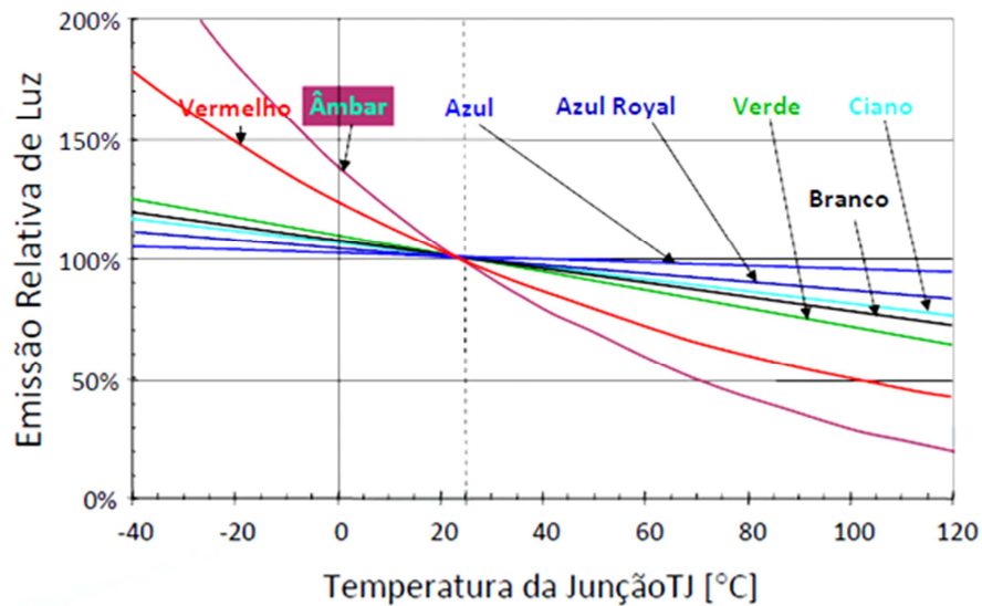
Figura 36 – Relação entre a temperatura dos LEDs e o fluxo luminoso emitido.
