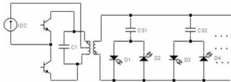
Figura 53 – Equalização com conversor push-pull ressonante e capacitores de saída (BADDELA e ZINGER, 2004).
