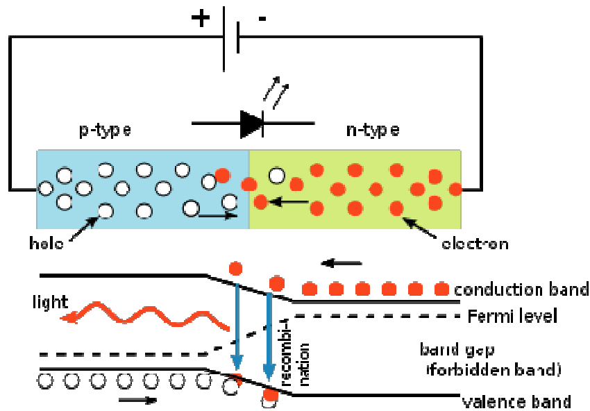
Figura 32 – Esquema de funcionamento de um LED.
