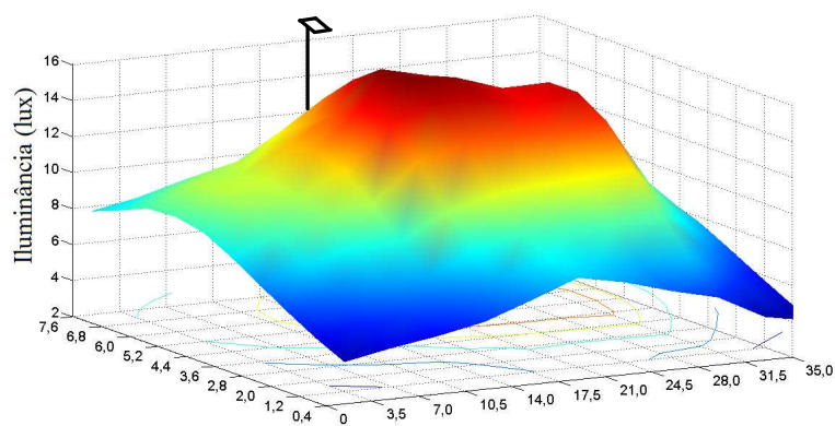
Figura 103 – Iluminância ponto a ponto com luminárias LED C1. Unidades no plano em metros.
