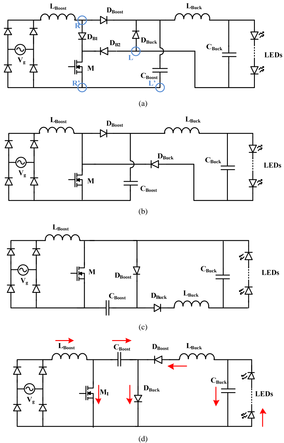
Figura 64 – Aplicação da técnica de integração ao dos conversores boost buck em cascata.
