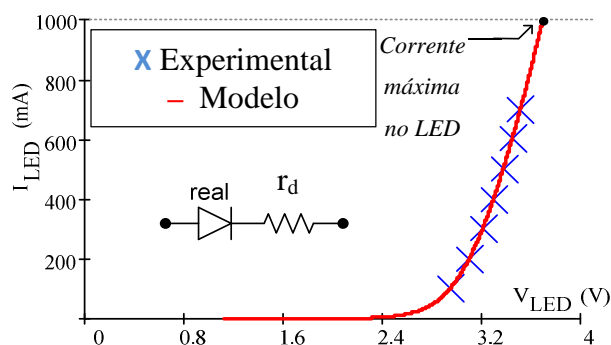
Figura 37 – Modelo elétrico de um LED de potência branco (ALMEIDA, et al., 2011c).
