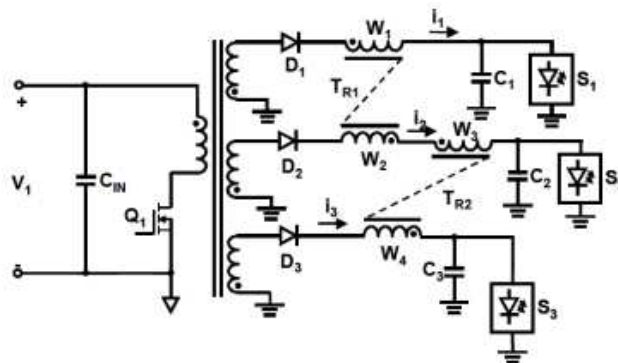
Figura 54 – Equalização com transformadores de balanceamento de corrente (HU e JOVANOVIĆ, 2011).
