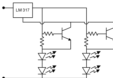
Figura 51 – Equalizador de corrente linear circuito integrado regulador monolítico.
