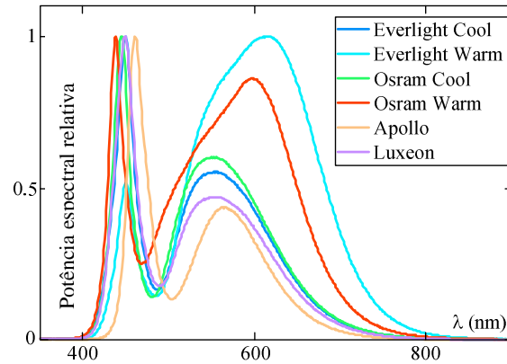
Figura 40 – Distribuição espectral de potência de diversos LEDs HP, normalizadas (RODRIGUES, et al., 2011c).
