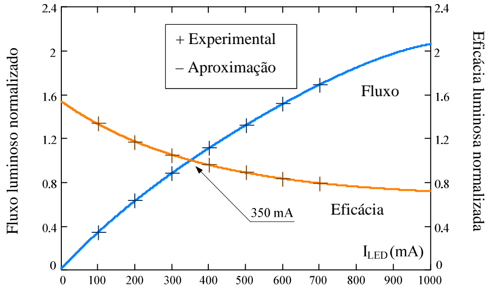
Figura 44 – Variação do fluxo e da eficácia luminosa do LED com variações da corrente direta (ALMEIDA, et al., 2011b).
