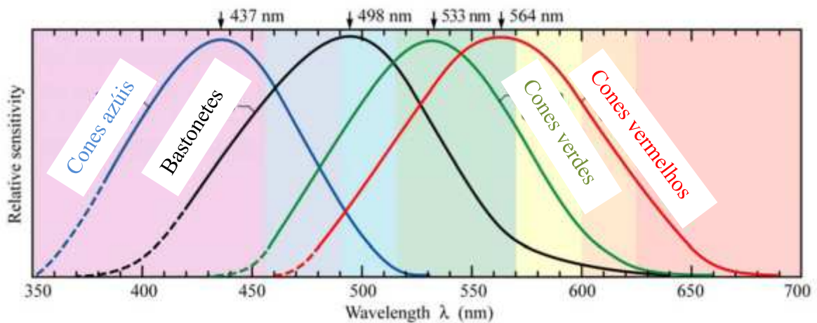
Figura 20 – Curva de sensibilidade relativa normalizada dos cones e dos bastonetes (SCHUBERT, 2003).
