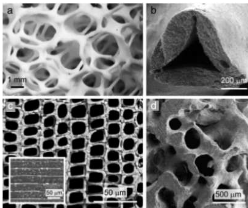
Figura 3 – Microestruturas de cerâmica macroporosa produzidas através da técnica de replica. (a) Estrutura de célula aberta à base de alumina obtida usando gabaritos de esponja de poliuretano, [85] (b) Detalhe de um suporte de uma cerâmica celular produzida a partir de esponjas poliméricas, ilustrando as falhas típicas formadas na pirólise do gabarito orgânico, [86] (c) Visão transversal de um SiC altamente orientado [83,87,88] (d) hidroxiapatita macroporosa obtida de uma estrutura de coral, [87].
