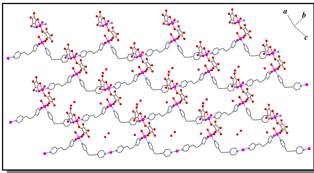
Figura 67 Extensão bidimensional do polímero \{[Mn_2(BPP)_2(C_5O_5)_2(H_2O)_4].3H_2O\}_n ( 10 ).
