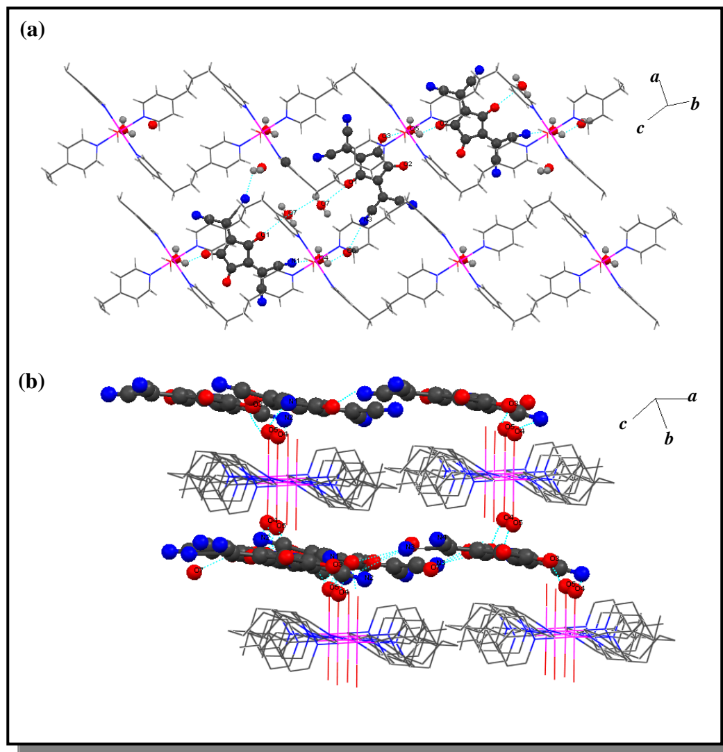
Figura 90 Representação do arranjo supramolecular de (15): (a) bidimensional e (b) tridimensional.
