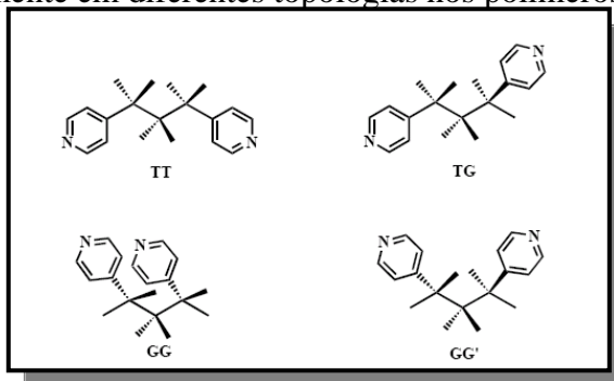
Figura 9 Diferentes conformações do ligante nitrogenado BPP.
