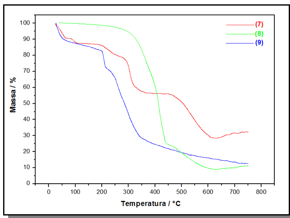
Figura 49 Curva termogravimétrica para os compostos (7), (8) e (9).
