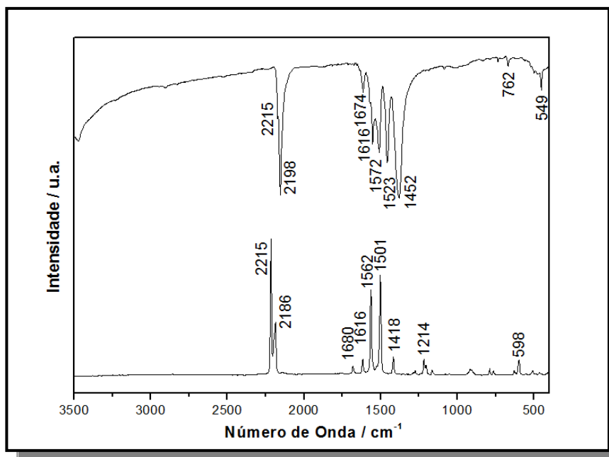
Figura 78 Espectros IV e Raman obtidos para o sal croconato violeta, K_2CV \cdot 2,5H_2O .
