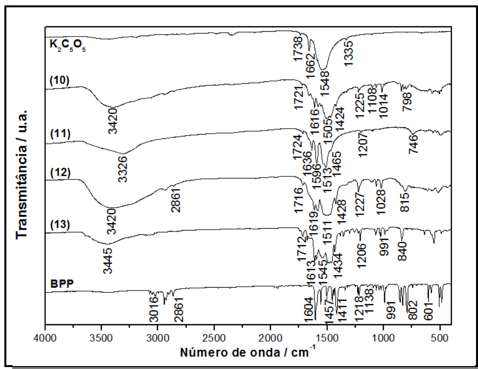
Figura 63 Espectros IV dos compostos (10) , (11) , (12) e (13) , bem como de seus precursores BPP e \text{K}_2\text{C}_5\text{O}_5 .
