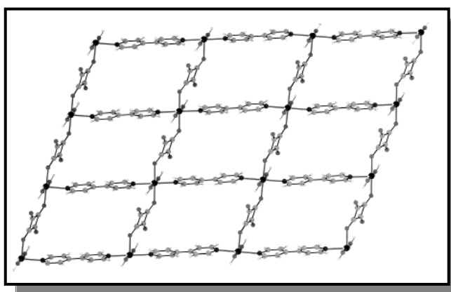
Figura 31 Visualização do polímero 2-D descrito na literatura, entre esquarato e o ligante espaçador 4,4'-bipiridina.
