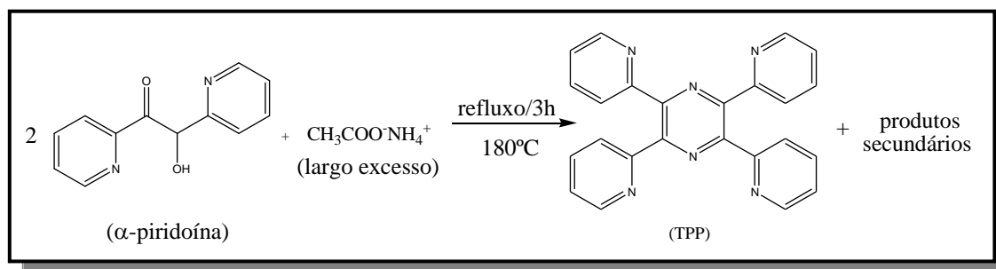
Figura 13 Representação esquemática da síntese do ligante TPP.
