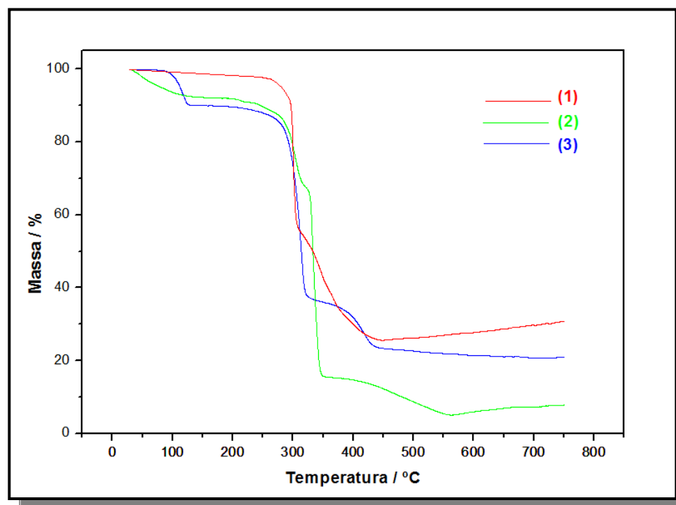
Figura 21 Curvas termogravimétricas para os compostos [Co(MBP) 2 (C 4 O 4 )]( 1 ), [Ni(MBP) 3 ](C 4 O 4 ).3H 2 O ( 2 ) e {[Cu 2 (MBP) 2 (C 4 O 4 ) 2 (H 2 O) 4 ]} n ( 3 ).
