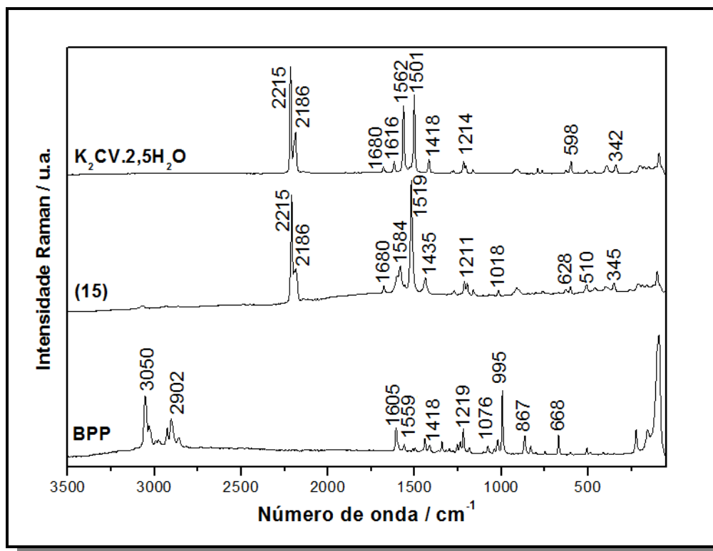
Figura 85 Espectros Raman dos precursores K_2CV.2,5H_2O e BPP e do composto \{[Mn(BPP)_2(H_2O)_2](CV)^{2-}.2H_2O\}_n (15).
