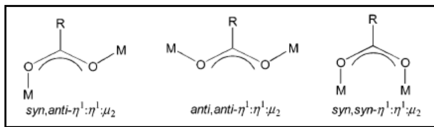
Figura 69 Representação de alguns dos modos de coordenação ao sítio metálico possíveis para carboxilatos.
