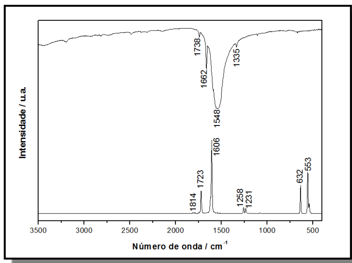
Figura 48 Espectros IV e Raman obtidos para o sal croconato de potássio ( K_2C_5O_5 ).
