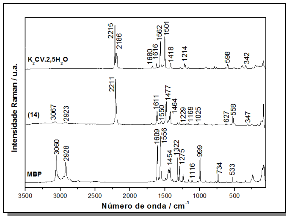
Figura 81 Espectros Raman para o precursoros K_2CV.2,5H_2O e MBP e para o complexo [Co(MBP)_2(CV)] ( 14 ).
