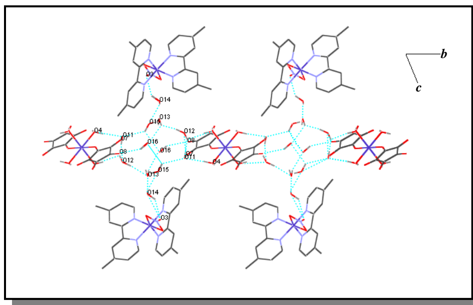
Figura 56 Extensão através de ligações de hidrogênio no complexo (7).
