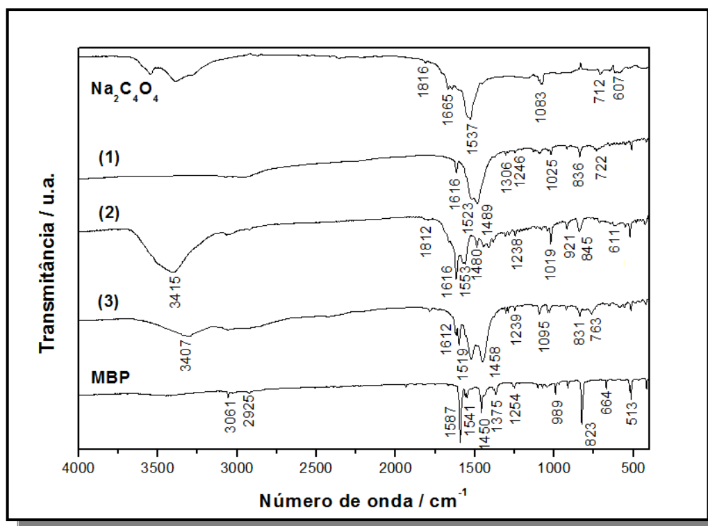
Figura 23 Espectros de absorção na região do infravermelho para os compostos [\text{Co}(\text{MBP})_2(\text{C}_4\text{O}_4)] (1), [\text{Ni}(\text{MBP})_3](\text{C}_4\text{O}_4) \cdot 3\text{H}_2\text{O} (2) e \{[\text{Cu}_2(\text{MBP})_2(\text{C}_4\text{O}_4)_2(\text{H}_2\text{O})_4]\}_n (3), bem como para os ligantes MBP e \text{Na}_2\text{C}_4\text{O}_4 .
