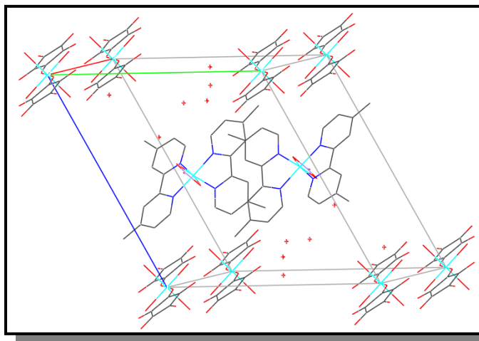
Figura 55 Representação da célula unitária do complexo (7). Os átomos de hidrogênio foram omitidos.
