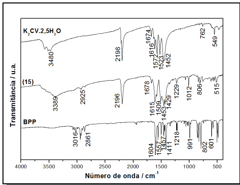
Figura 84 Espectros na região do infravermelho dos precursores K_2CV.2,5H_2O e BPP e do composto \{[Mn(BPP)_2(H_2O)_2](CV).2H_2O\}_n ( 15 ).
