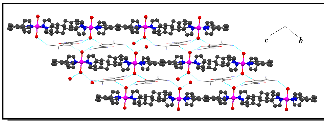
Figura 88 Extensão bidimensional do polímero de coordenação ( 15 ) ao longo da diagonal do plano (100)
