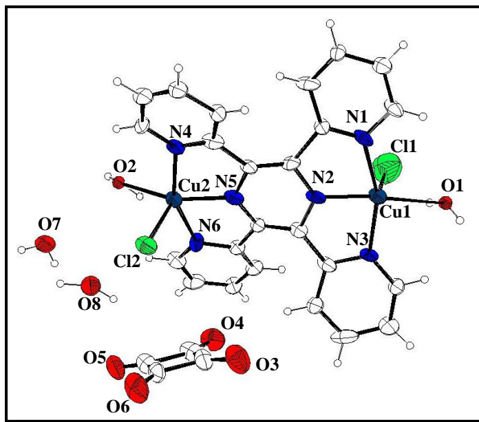
Figura 38 Representação da unidade assimétrica do composto [\text{Cu}_2(\text{TPP})(\text{H}_2\text{O})_2\text{Cl}_2](\text{C}_4\text{O}_4)\cdot 2\text{H}_2\text{O} ( 6 ).
