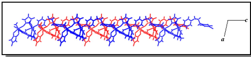
Figura 74 Visão lateral das camadas onduladas 2-D interpenetradas de (10) .
