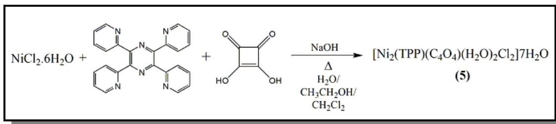
Figura 18 Esquema da metodologia de síntese do composto [\text{Ni}_2(\text{TPP})(\text{C}_4\text{O}_4)(\text{H}_2\text{O})_2\text{Cl}_2]7\text{H}_2\text{O} (5).
