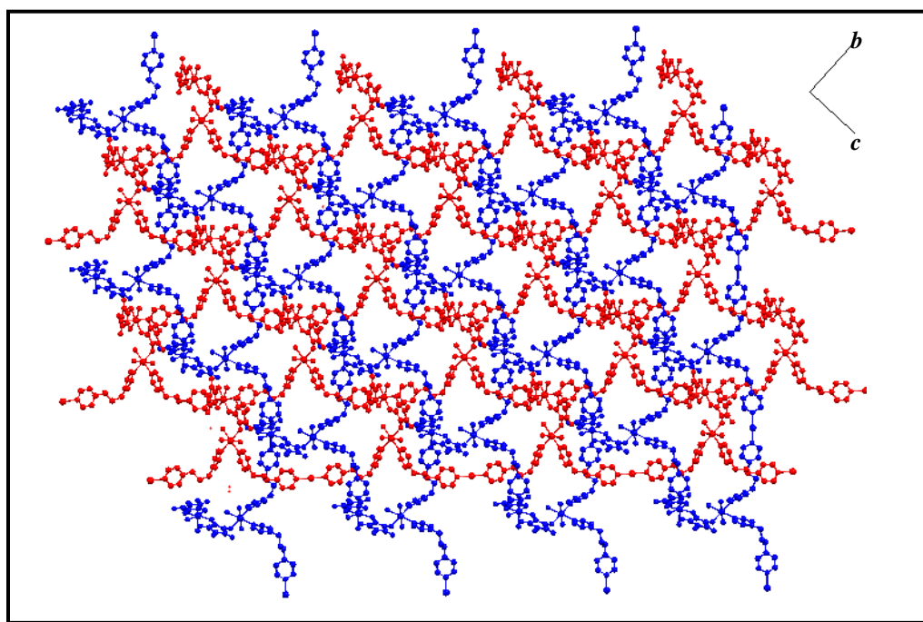
Figura 73 Representação evidenciando a interpenetração paralela de duas redes poliméricas 2-D do tipo (6,3) de (10) .
