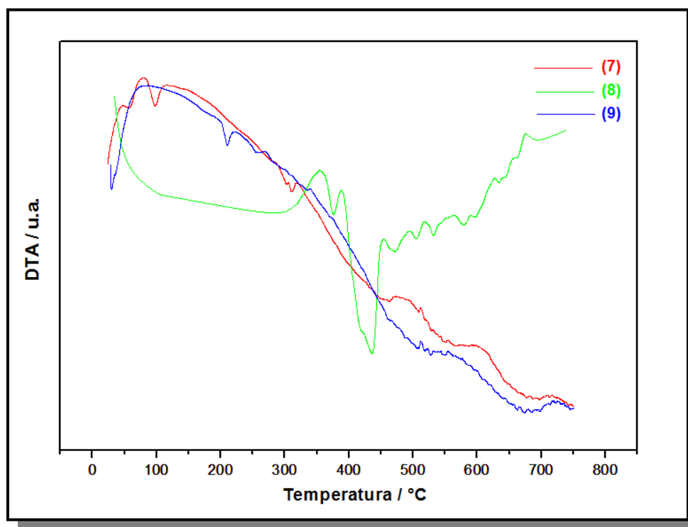
Figura 50 Curvas DTA para os compostos (7), (8) e (9).
