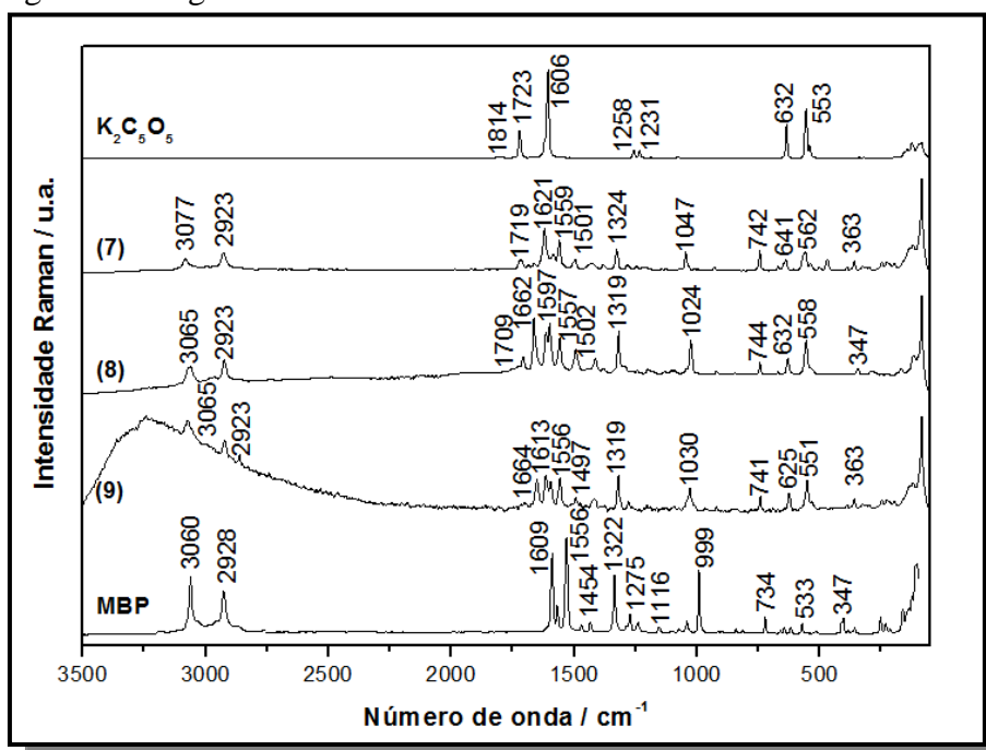
Figura 52 Espectros Raman dos obtidos para os compostos (7), (8) e (9) e de seus precursores MBP e \text{K}_2\text{C}_5\text{O}_5 .
