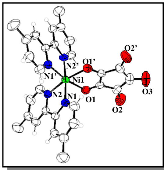
Figura 58 Representação da estrutura cristalina e molecular do complexo [\text{Ni}(\text{MBP})_2(\text{C}_5\text{O}_5)] ( 8 ).
