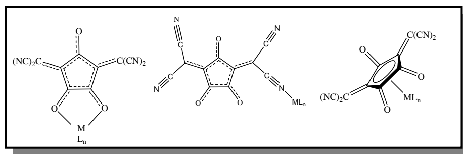
Figura 5 Diferentes modos de coordenação ao sítio metálico do ligante croconato violeta .
