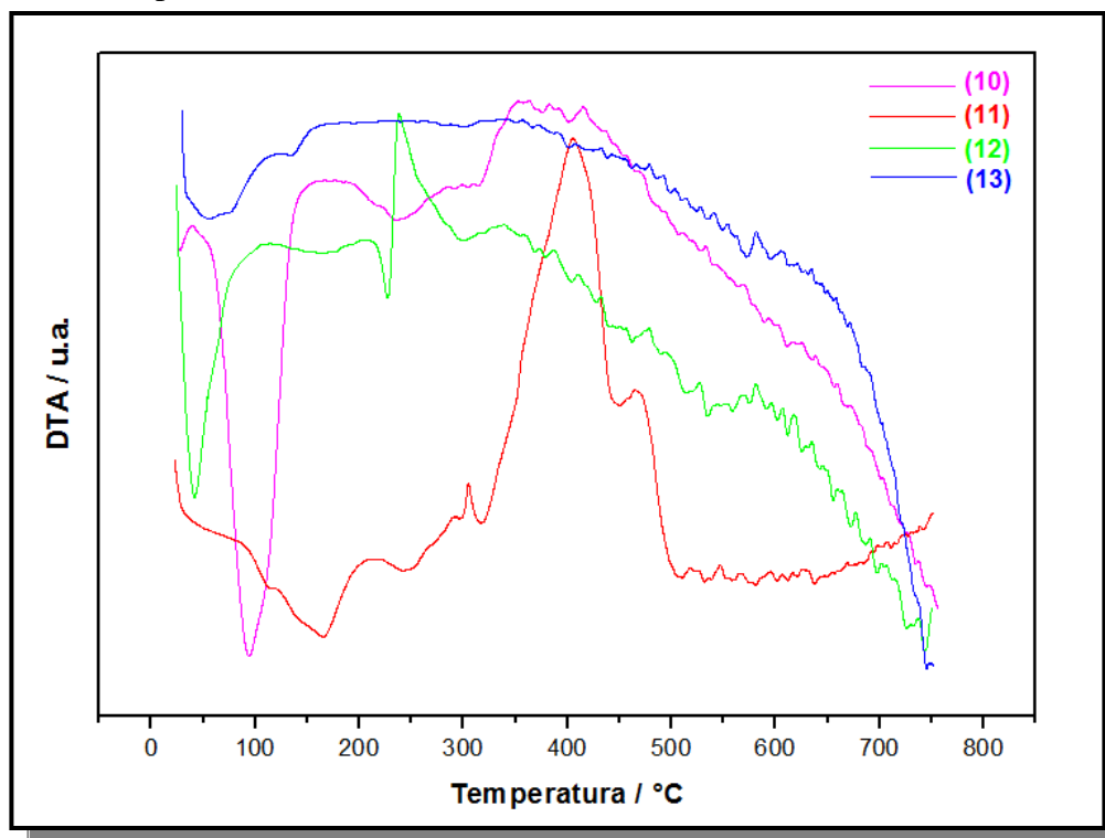
Figura 62 Curva DTA dos compostos (10) , (11) , (12) e (13) .
