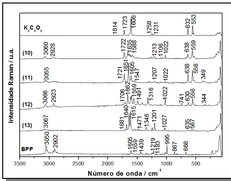
Figura 64 Espectros Raman dos compostos (10), (11), (12) e (13), bem como de seus precursores BPP e K_2C_5O_5 .
