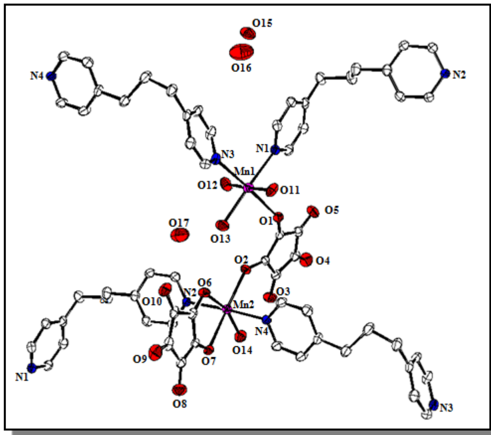
Figura 66 Estrutura cristalina do \{[Mn_2(BPP)_2(C_5O_5)_2(H_2O)_4] \cdot 3H_2O\}_n ( 10 ).
