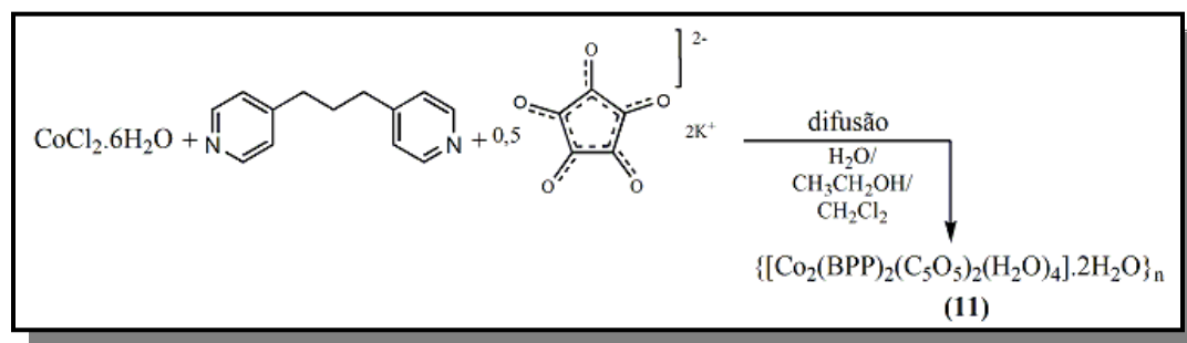
Figura 45 Esquema da rota sintética de obtenção de \{[\text{Co}_2(\text{BPP})_2(\text{C}_5\text{O}_5)_2(\text{H}_2\text{O})_4]\cdot 2\text{H}_2\text{O}\}_n (11).
