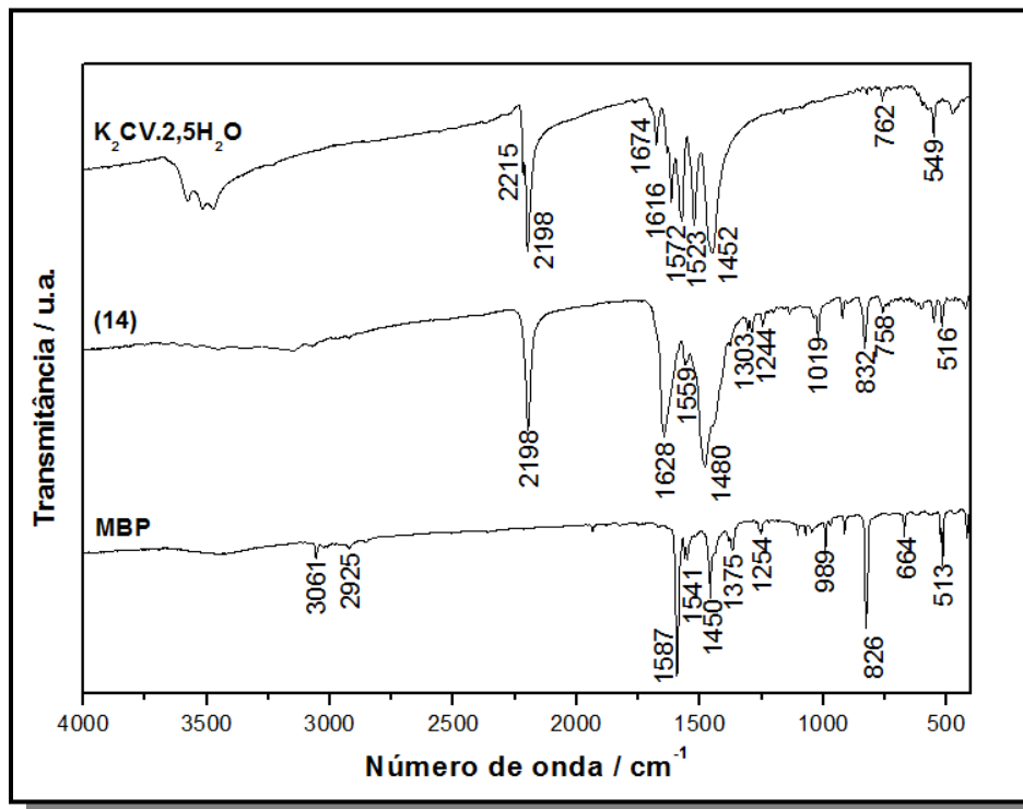
Figura 80 Espectros de Infravermelho dos ligantes K_2CV.2,5H_2O e MBP e do complexo [Co(MBP)_2(CV)] (14) .
