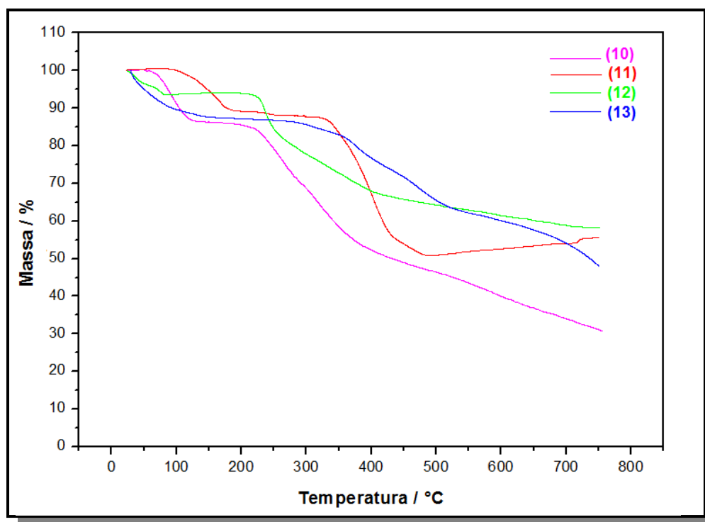
Figura 61 Curva termogravimétrica para os compostos de coordenação ( 10 ), ( 11 ), ( 12 ) e ( 13 ).
