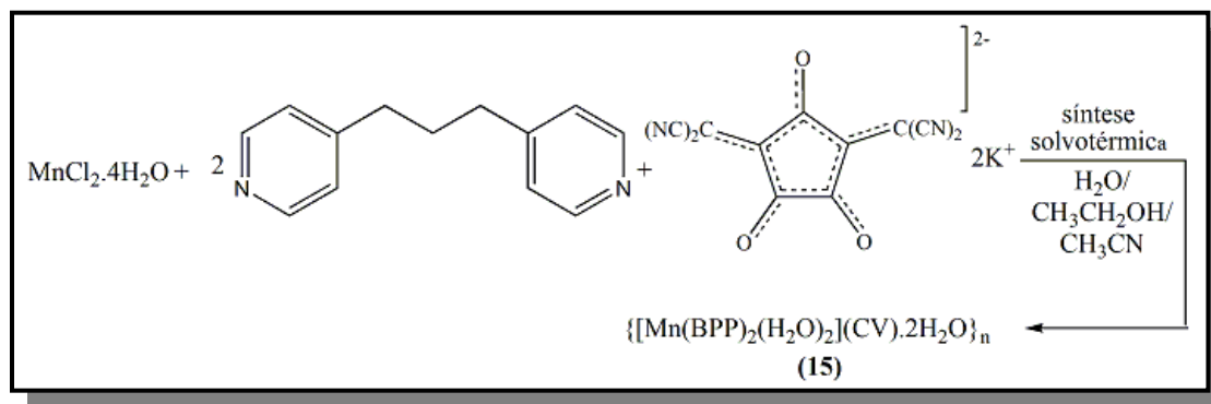
Figura 77 Metodologia sintética de \{[\text{Mn}(\text{BPP})_2(\text{H}_2\text{O})_2](\text{CV})^{2-}\cdot 2\text{H}_2\text{O}\}_n ( 15 ).
