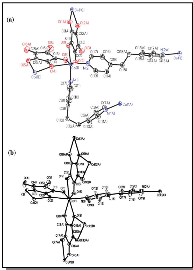
Figura 71 Representação da estrutura cristalina dos compostos descritos na literatura: (a) [\text{Co}(\text{BPE})(\text{C}_5\text{O}_5)] e (b) \{[\text{Cd}_2(\text{C}_5\text{O}_5)_2(4,4'\text{-bipy})(\text{H}_2\text{O})]\cdot\text{H}_2\text{O}\}_n .
