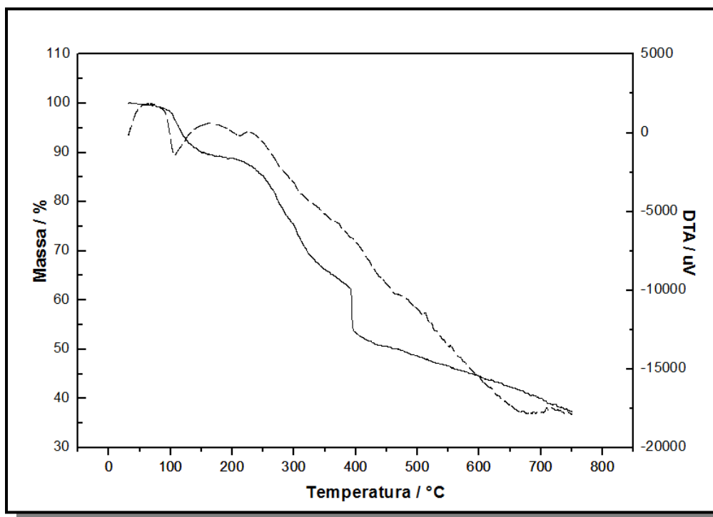
Figura 83 Curvas TG e DTA para o composto \{[\text{Mn}(\text{BPP})_2(\text{H}_2\text{O})_2](\text{CV})^{2-} \cdot 2\text{H}_2\text{O}\}_n ( 15 ).
