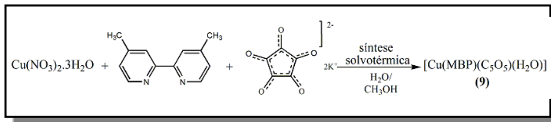
Figura 43 Esquema da metodologia de síntese do composto [Cu(MBP)(C 5 O 5 )(H 2 O)] (9).
