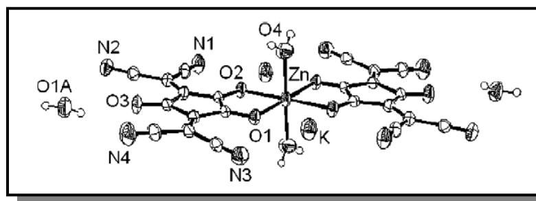
Figura 6 Estrutura molecular do complexo K_2[Zn(CV)_2(H_2O)_2] \cdot 2H_2O .
