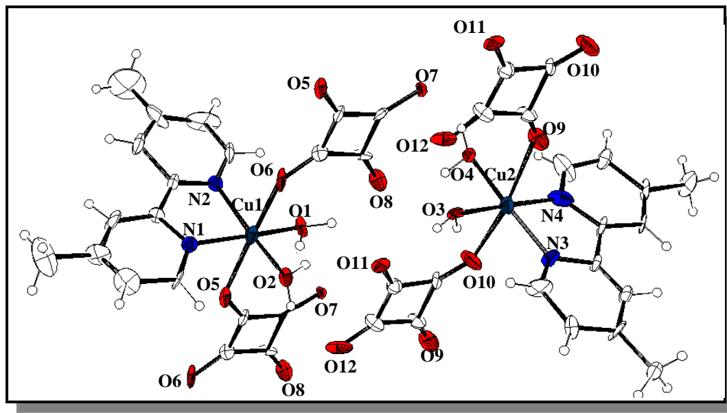
Figura 28 Estrutura molecular do complexo \{[Cu_2(MBP)_2(C_4O_4)_2(H_2O)_4]\}_n ( 3 ).
