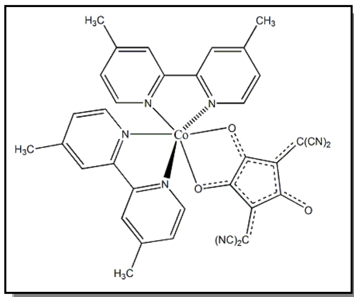
Figura 82 Proposta estrutural para o composto [Co(MBP) 2 (CV)] (14).
