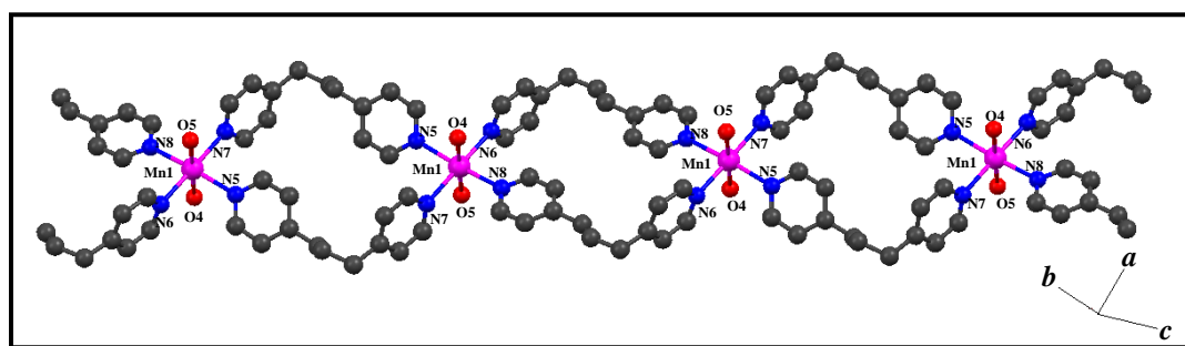
Figura 87 Extensão unidimensional (1-D) do polímero de coordenação [\text{Mn}(\text{BPP})_2(\text{H}_2\text{O})_2](\text{CV}) \cdot 2\text{H}_2\text{O} ( 15 ).
