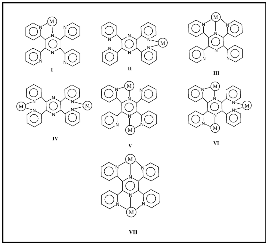
Figura 11 Modos de coordenação observados para o ligante TPP.
