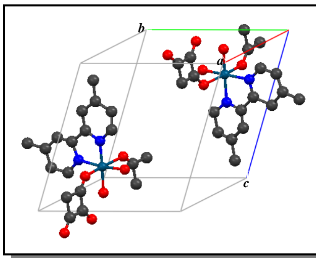
Figura 29 Visualização da célula unitária do composto ( 3 ). Os átomos de hidrogênio não foram representados.
