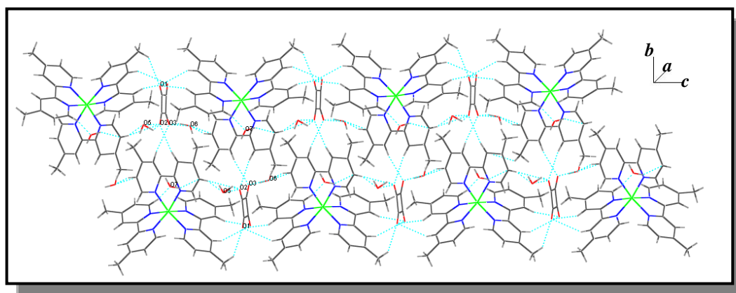
Figura 27 Arranjo bidimensional através de ligações de hidrogênios e dipolo-dipolo induzido do composto (2).
