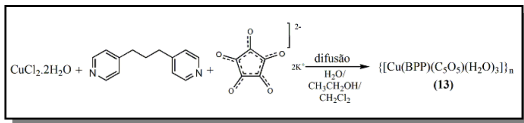
Figura 47 Representação esquemática da síntese de \{[\text{Cu}(\text{BPP})(\text{C}_5\text{O}_5)(\text{H}_2\text{O})_3]\}_n ( 13 ).
