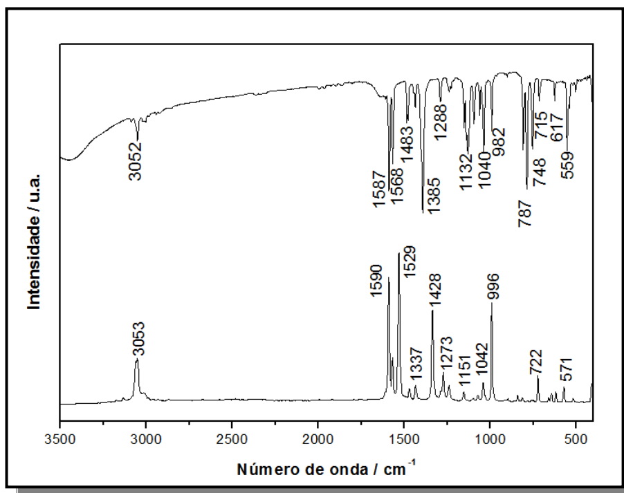
Figura 20 Espectros IV e Raman obtidos para o ligante TPP
