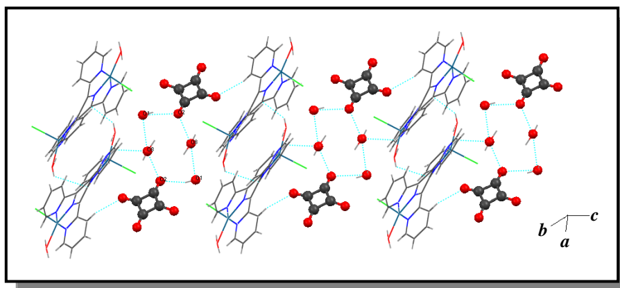
Figura 39 Visualização do hexâmero formado através de ligações de hidrogênio em (6).
