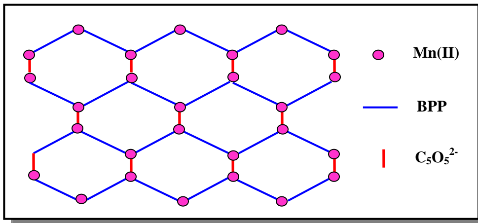
Figura 68 Representação dos caminhos fechados de (10) semelhantes à colméia de abelha distorcida.
