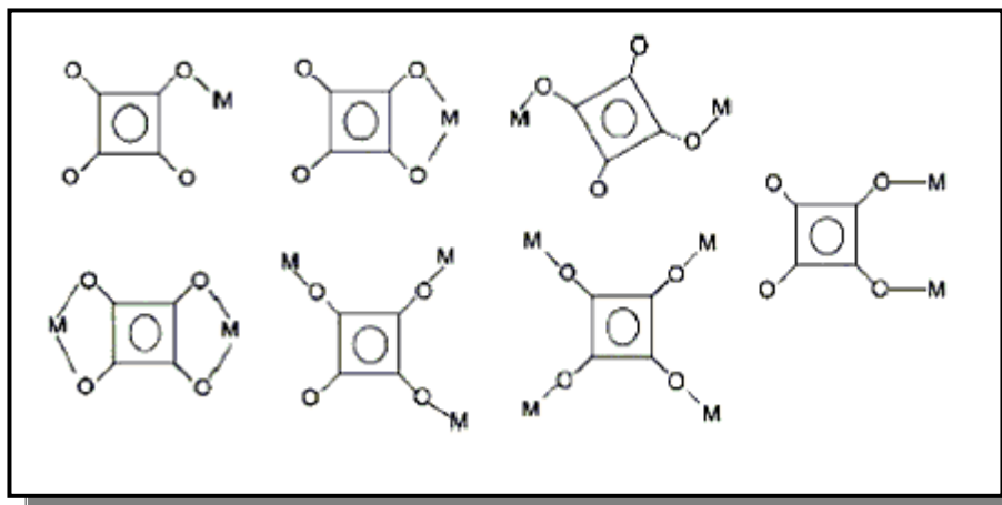
Figura 2 Diferentes modos de coordenação ao sítio metálico do ligante esquarato.
