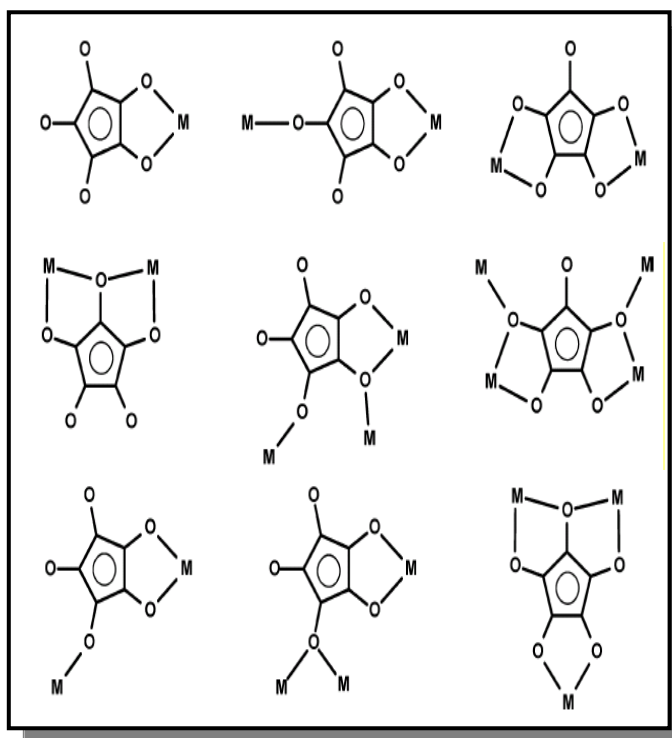
Figura 3 Diferentes modos de coordenação ao sítio metálico do ligante croconato.
