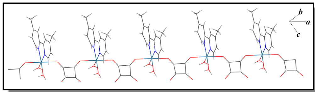
Figura 30 Estrutura cristalina do polímero de coordenação (3) estendido em 1-D pelo ligante esquarato ao longo do eixo cristalográfico a .
