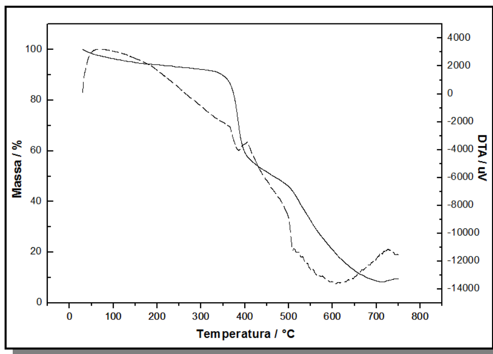
Figura 79 Curvas TG e DTA do composto [\text{Co}(\text{MBP})_2(\text{CV})] ( 14 ).
