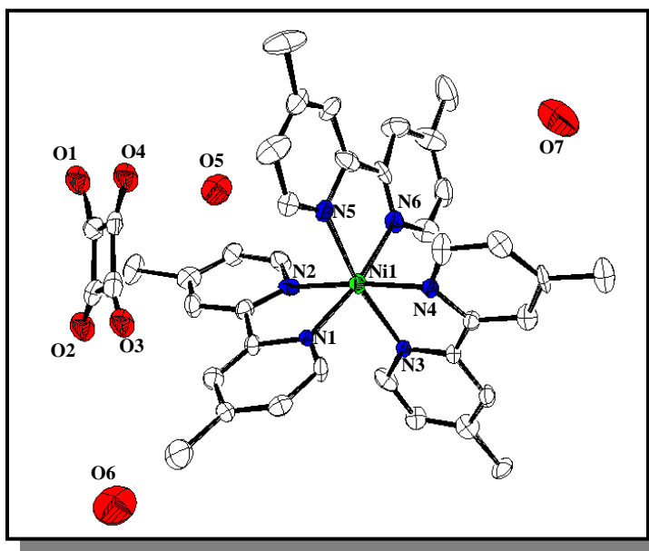
Figura 26 Representação da unidade assimétrica do composto [\text{Ni}(\text{MBP})_3](\text{C}_4\text{O}_4) \cdot 3\text{H}_2\text{O} ( 2 ). Os átomos de hidrogênio não foram representados.
