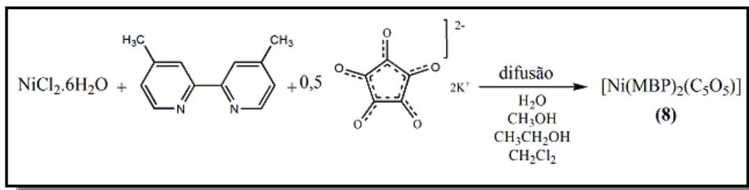
Figura 42 Esquema da metodologia de síntese do composto [\text{Ni}(\text{MBP})_2(\text{C}_5\text{O}_5)] (8).
