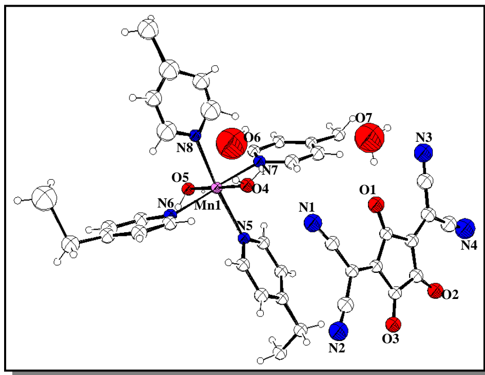
Figura 86 Representação da unidade assimétrica do polímero de coordenação \{[Mn(BPP)_2(H_2O)_2](CV) \cdot 2H_2O\}_n ( 15 ).
