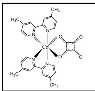
Figura 25 Representação da proposta estrutural para o composto [\text{Co}(\text{MBP})_2(\text{C}_4\text{O}_4)] ( 1 ).
