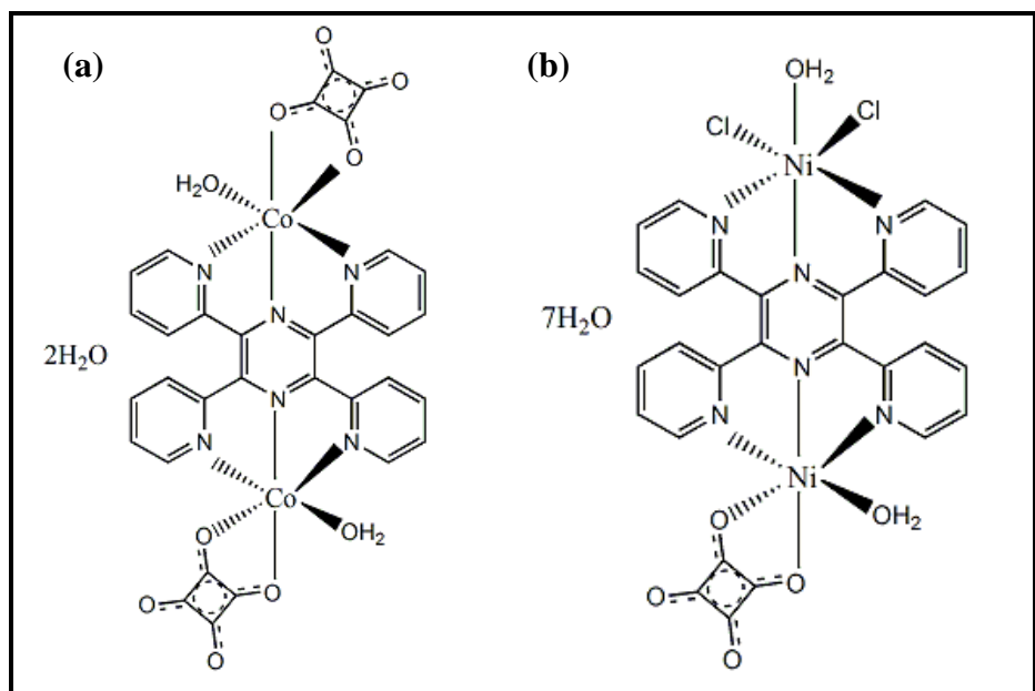
Figura 37 Representação esquemática das propostas estruturais para os compostos: (a) [\text{Co}_2(\text{TPP})(\text{C}_4\text{O}_4)_2(\text{H}_2\text{O})_2] \cdot 2\text{H}_2\text{O} (4) e (b) [\text{Ni}_2(\text{TPP})(\text{C}_4\text{O}_4)(\text{H}_2\text{O})_2\text{Cl}_2] \cdot 7\text{H}_2\text{O} (5) .
