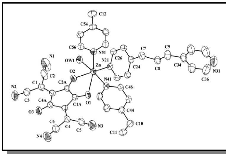
Figura 10 Projeção da unidade assimétrica do polímero {[Zn( \mu -BPP)(BPP)(CV)(H 2 O)].H 2 O} n
