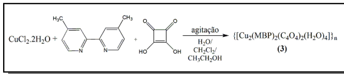
Figura 16 Esquema da metodologia de síntese do composto \{[\text{Cu}_2(\text{MBP})_2(\text{C}_4\text{O}_4)_2(\text{H}_2\text{O})_4]\}_n (3).
