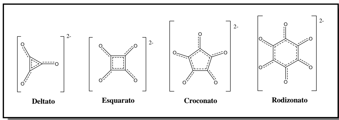
Figura 1 Representação esquemática das estruturas dos íons oxocarbonos: deltato ( C_3O_3^{2-} ), esquarato ( C_4O_4^{2-} ), croconato ( C_5O_5^{2-} ) e rodizonato ( C_6O_6^{2-} ).
