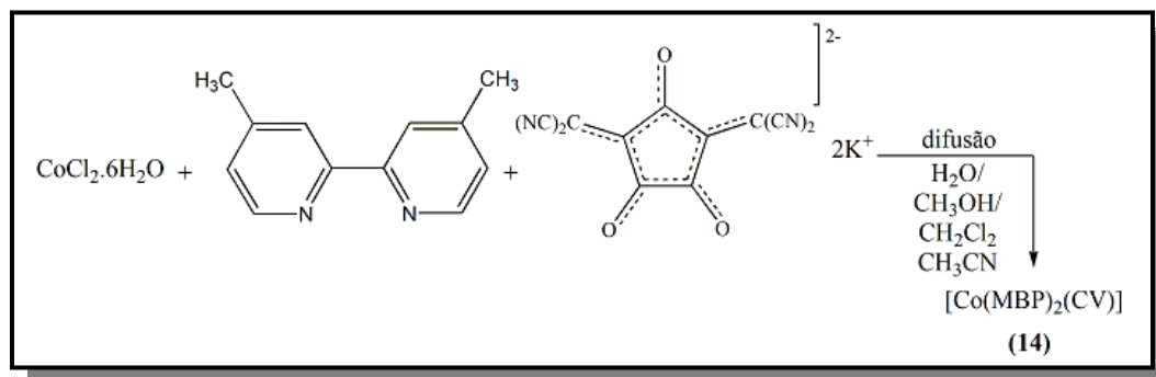
Figura 76 Esquema da metodologia de síntese do composto [\text{Co}(\text{MBP})_2(\text{CV})] (14).
