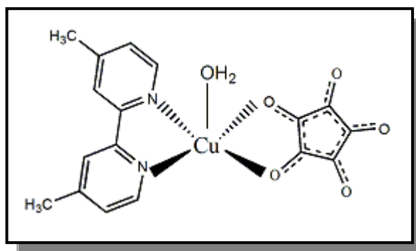
Figura 53 Proposta estrutural para o composto [\text{Cu}(\text{MBP})(\text{C}_5\text{O}_5)(\text{H}_2\text{O})] (9) .
