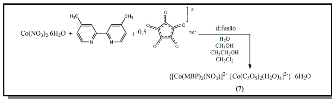
Figura 41 Esquema da metodologia de síntese do composto \{[\text{Co}(\text{MBP})_2(\text{NO}_3)]^{2+} \cdot [\text{Co}(\text{C}_5\text{O}_5)_2(\text{H}_2\text{O})_4]^{2-}\} \cdot 6\text{H}_2\text{O} (7).
