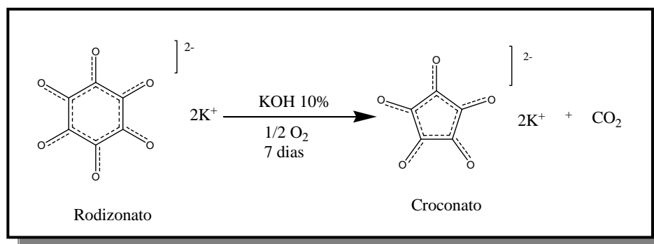
Figura 40 Representação esquemática da síntese do Croconato de Potássio.
