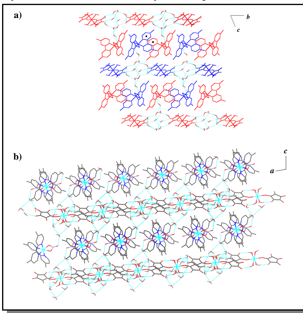
Figura 57 Extensão do arranjo supramolecular bidimensional de (7) ao longo do eixo cristalográfico c , (a) visualização ao longo do eixo cristalográfico a e (b) visualização ao longo de b .
