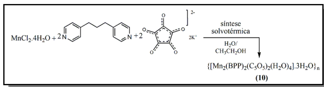
Figura 44 Esquema da metodologia de síntese do composto \{[\text{Mn}_2(\text{BPP})_2(\text{C}_5\text{O}_5)_2(\text{H}_2\text{O})_4].3\text{H}_2\text{O}\}_n (10).
