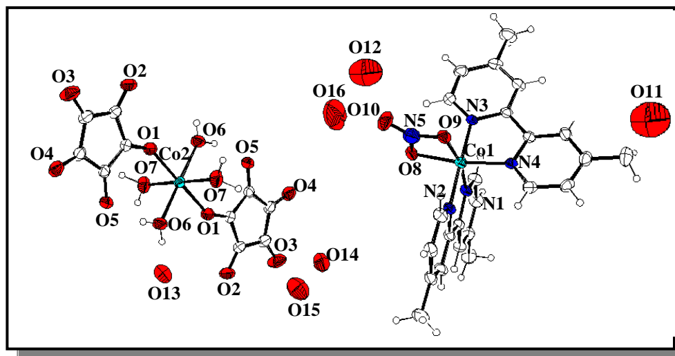
Figura 54 Representação da estrutura cristalina e molecular do complexo \{[Co(MBP)_2(NO_3)]^{2+} \cdot [Co(C_5O_5)_2(H_2O)_4]^{2-}\} \cdot 6H_2O (7). Os hidrogênios das moléculas de H_2O não foram representados.
