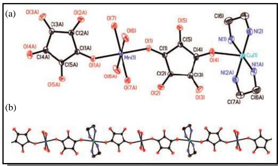
Figura 70 Representação da unidade assimétrica em (a), bem como da extensão unidimensional do polímero [\text{Cu}(\text{en})_2][\text{Mn}(\text{C}_5\text{O}_5)_2(\text{H}_2\text{O})_4] \cdot 2\text{H}_2\text{O} em (b), descrito na literatura.
