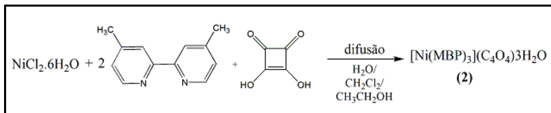
Figura 15 Esquema da metodologia de síntese do composto [\text{Ni}(\text{MBP})_3](\text{C}_4\text{O}_4)\cdot 3\text{H}_2\text{O} (2).
