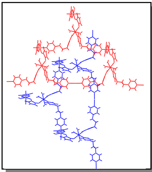
Figura 72 Representação revelando a interpenetração das unidades de construção presentes em diferentes redes poliméricas 2-D em (10) .
