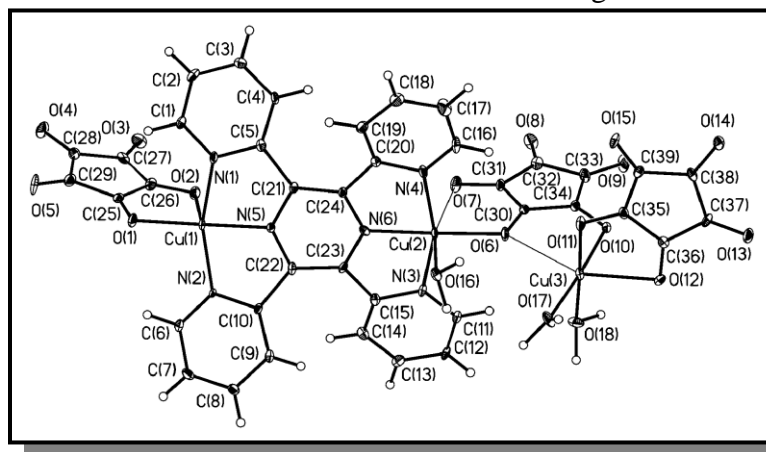
Figura 12 Estrutura molecular do bloco construtor [Cu_3(TPP)(C_5O_5)_3(H_2O)_3] .
