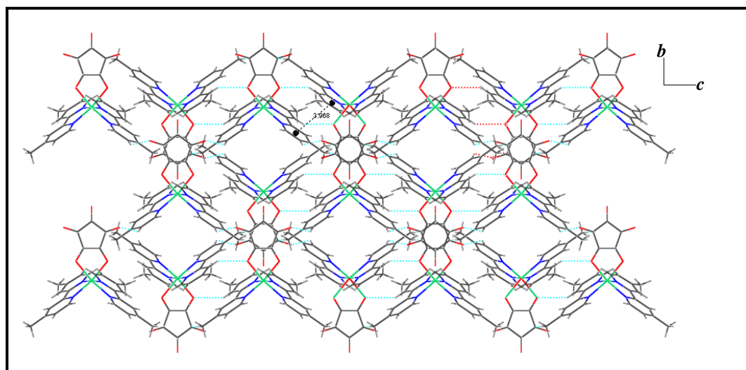
Figura 59 Extensão do arranjo supramolecular em ( 8 ) por empacotamento \pi ao longo do eixo cristalográfico c .
