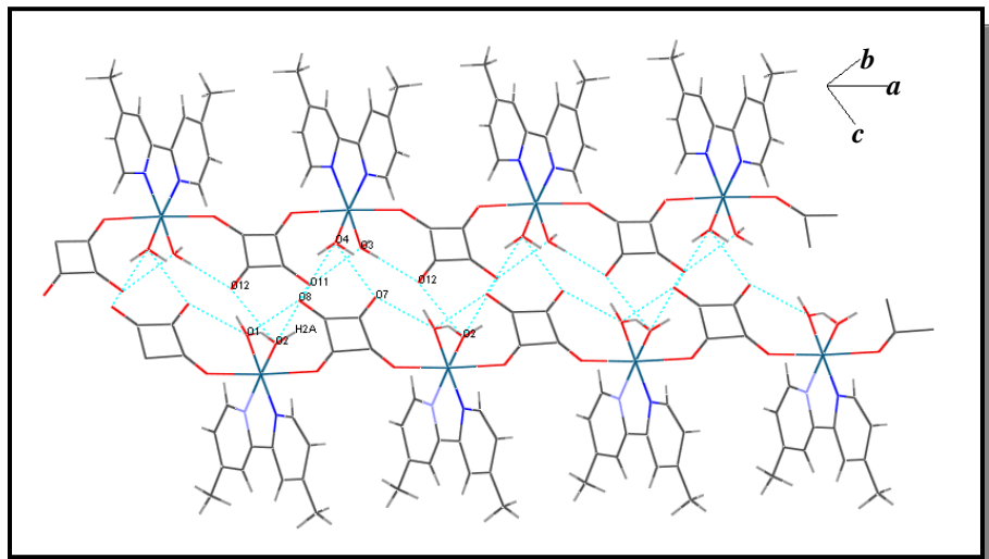
Figura 32 Extensão do arranjo supramolecular 2-D de (3) ao longo do eixo cristalográfico a .
