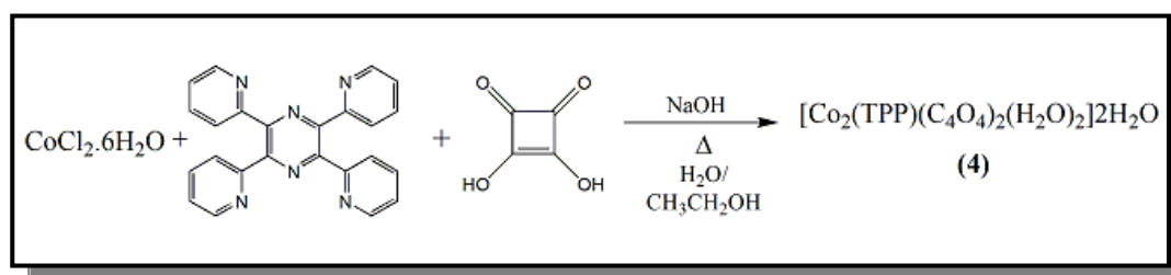
Figura 17 Esquema da metodologia de síntese do composto [\text{Co}_2(\text{TPP})(\text{C}_4\text{O}_4)_2(\text{H}_2\text{O})_2]2\text{H}_2\text{O} (4).
