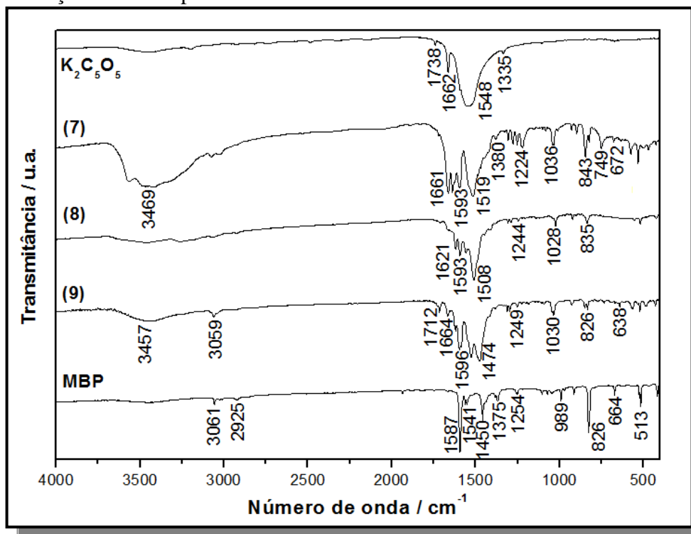
Figura 51 Espectros de absorção na região do infravermelho para os compostos (7), (8) e (9) e de seus precursores MBP e K_2C_5O_5 .
