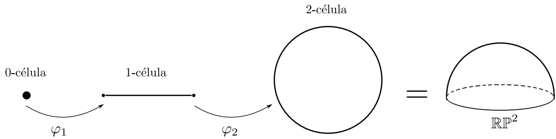
Figura 10 – Decomposição de \mathbb{R}P^2
