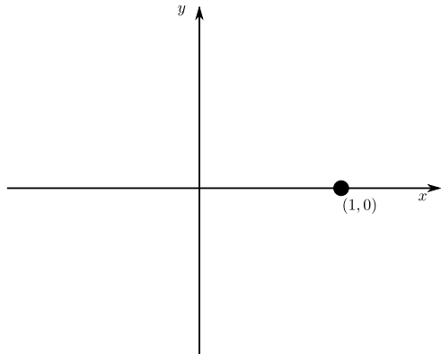
Figura 11 – Variedade estável S(L_1)
