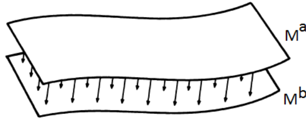
Figura 1 – Retrato por deformação
