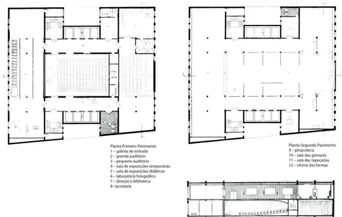
Figura 2. Planta baixa e transversal da adaptação do sete de abril, no Edifício Guilherme Guinle, 1950.
