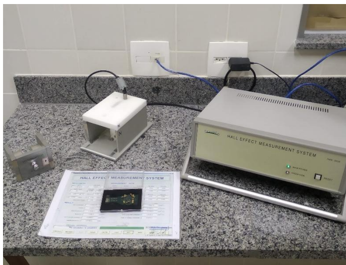
Figura 11. Sistema de medidas via efeito Hall Ecopia HMS-3000 utilizado neste trabalho.
