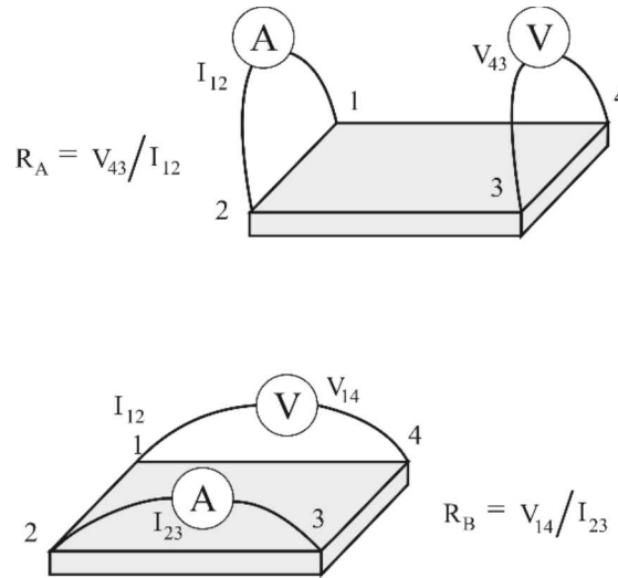
Figura 4. Esquema da medida de resistividade no método de van der Pauw. Imagem do próprio autor.
