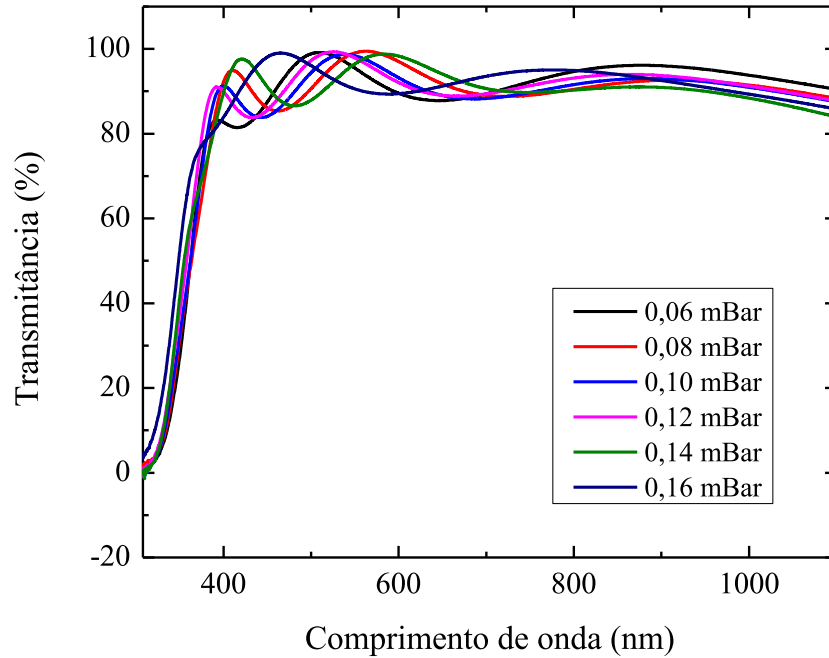
Figura 20. Espectros de transmitância óptica dos filmes finos de GZO para diferentes valores da pressão de trabalho.
