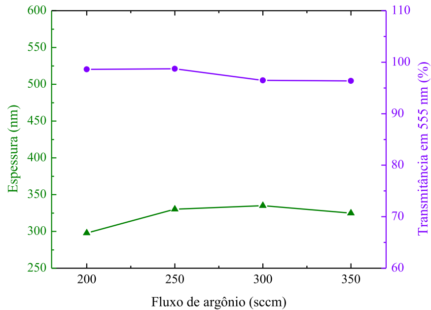
Figura 25. Espessura e transmitância ótica em função do fluxo de argônio utilizado.
