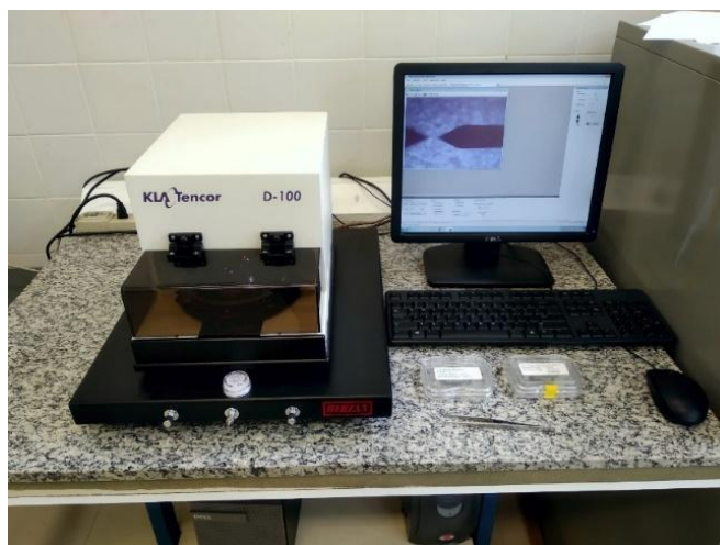
Figura 10. Perfilômetro KLA Tencor D-100 utilizado para aferir a espessura dos filmes de GZO.
