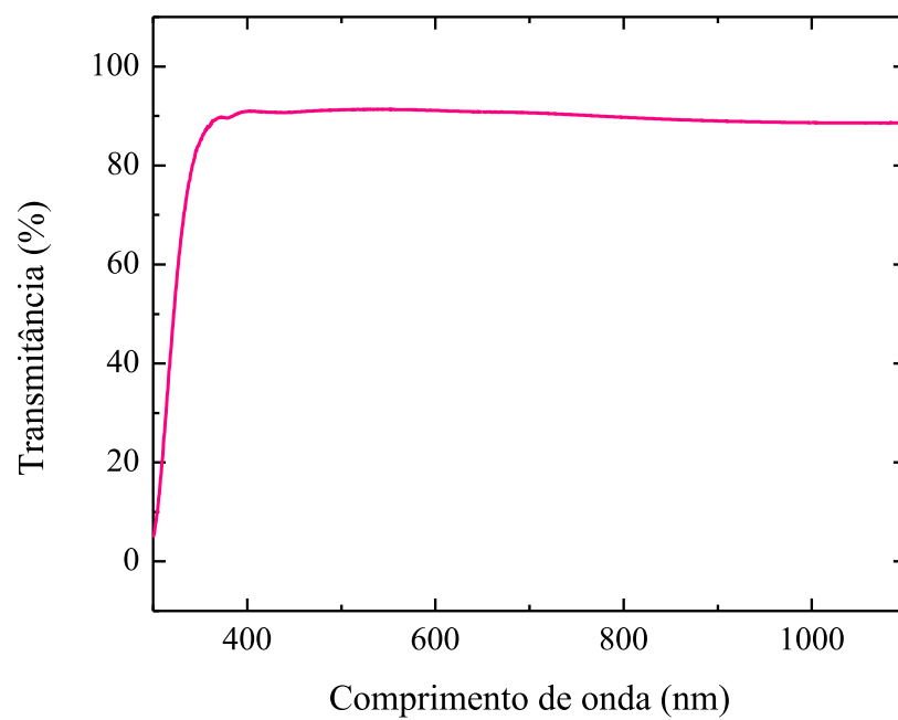
Figura 13. Transmissão de uma amostra de substrato de vidro em função do comprimento de onda da luz incidente.
