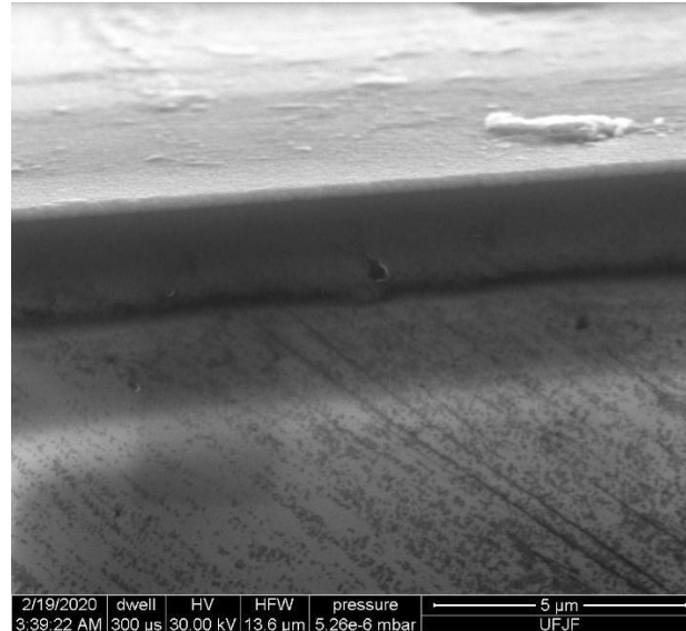
Figura 31. Imagem de microscopia eletrônica de varredura de um filme de GZO visto de perfil. A região mais clara é o filme pulverizado, em contraste com a região mais escura que é o substrato de vidro.
