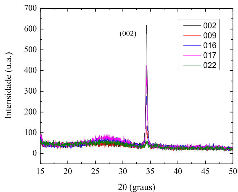
Figura 29. Difratomogramas de raios-X dos filmes finos de GZO obtidos com diferentes parâmetros de deposição.
